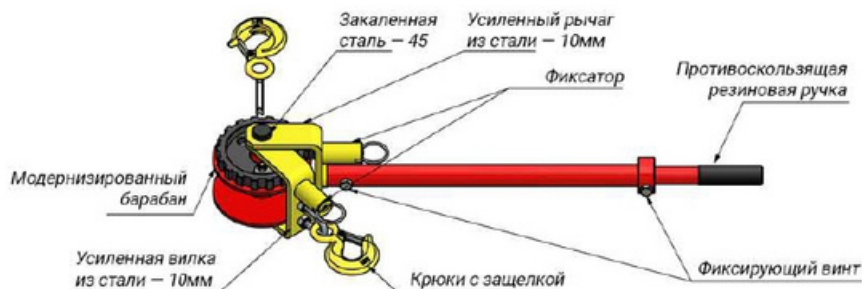
Рисунок 1. Устройство лебедки ручной рычажной модели ЛР.
