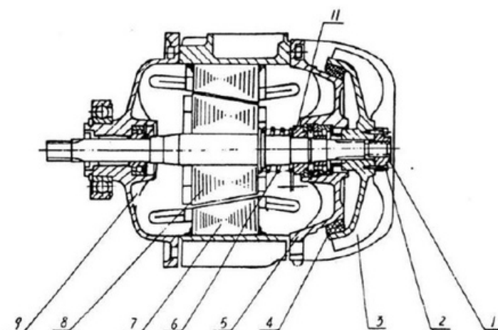
Рис.1 - Двигатель подъема для CDL 0,5-5 т.
