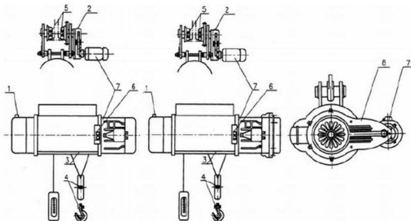
Рис.3 - Схема смазки тали CDL/MDL (чертеж тали схематичен)
