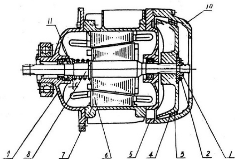
Рис.2 - Двигатель подъема для CDL 10 т.
