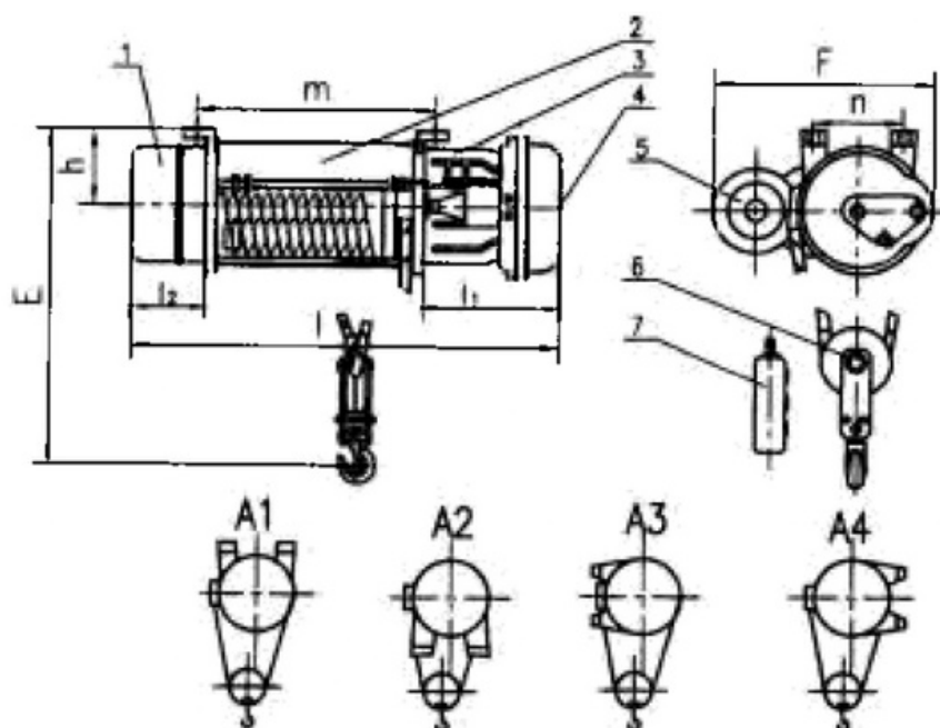
Рис.8 - Электрическая таль MD1 0.5 - 5 т, 6 - 36 м с жестким креплением 1. редуктор скорости подъемного механизма; 2. наматывающий барабан; 3. двигатель для перемещения в вертикальной плоскости; 4. регулятор тормоза; 5. двигатель малой скорости; 6. подъемный крюк; 7. кнопки нажимные
