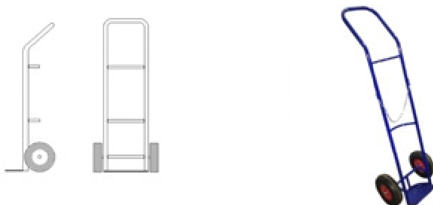
Рисунок 1. Тележка для бочек ГБ-1.
