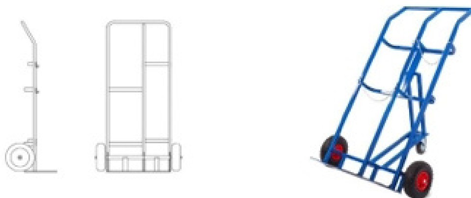
Рисунок 4. Тележка для бочек ТПК-П.
